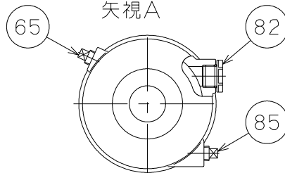
オイル室部 矢視A
