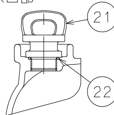
注水口部
