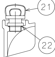
注水口部
