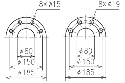
SUCTION FLANGE 吸込フランジ
